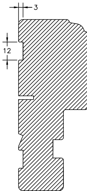
Kalfatring/ sløjfenot
