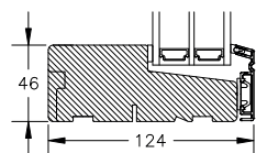
BUND- OG OVERKARM
