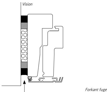
Vision fuges på træet.
