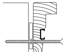
Montage af Vision topstyret vindue
